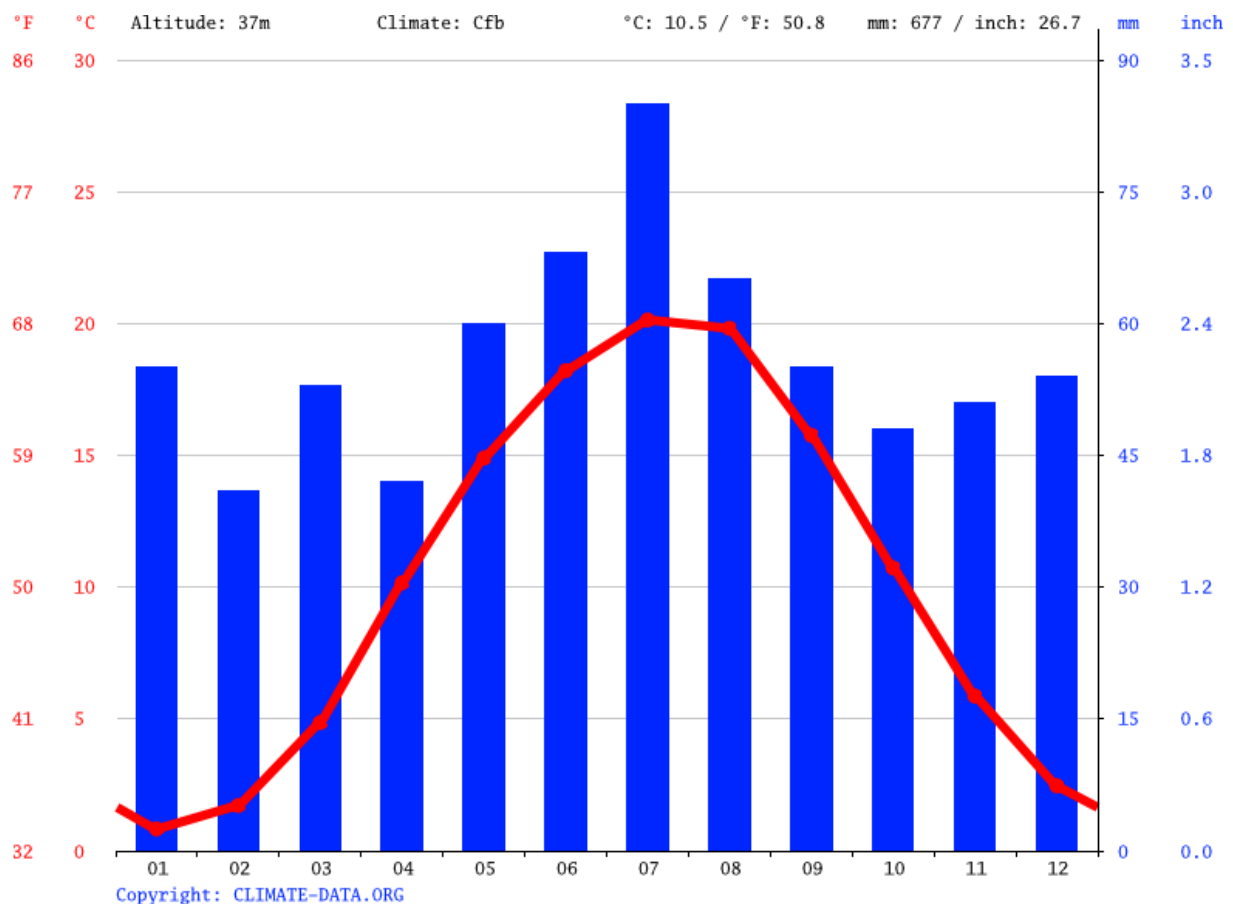
Abbildung 4: Klimadiagramm (Quelle: climate-data.org ).
